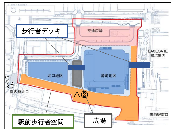
▲計画平面図
